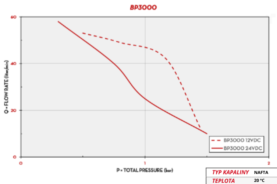
LAMELOVÝ ROTOR
