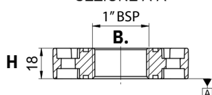
SEZIONE A-A
